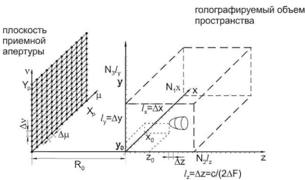
Рис.2. Схема синтеза оптических голограмм трехмерных объектов
