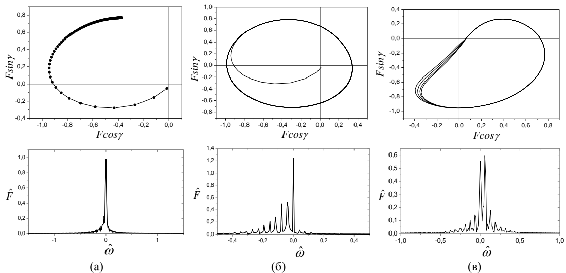
Рис. 3. Нестационарные характеристики электронно-волновой системы с предварительной модуляцией электронного потока. P_0 = -46 дБ.
