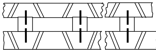
Рис.2. Схема фрагмента комплексированной волноводно-щелевой и вибраторной антенной решетки с излучателями, ортогональными по поляризации
