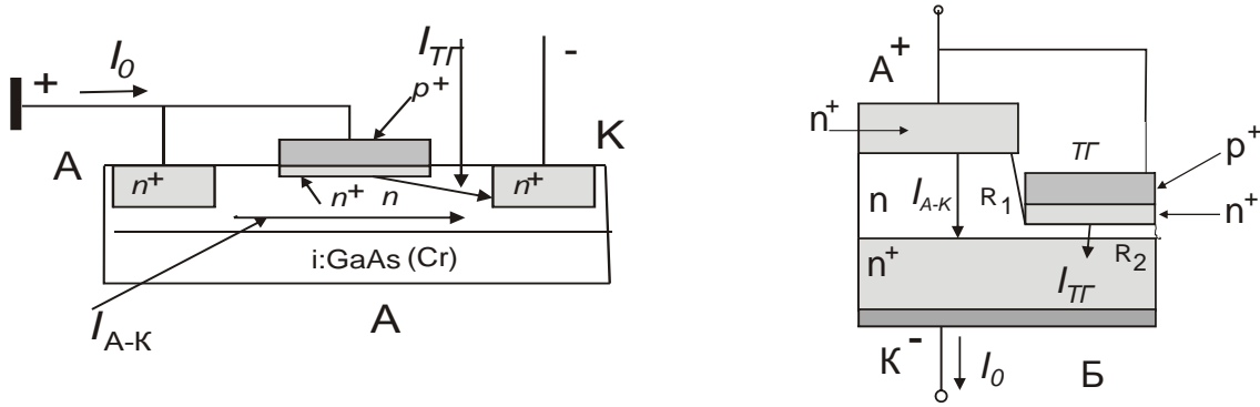
Рис. 1. Планарная структура диода с боковой p^+-n^+ ТГ на эпитаксиальной пленке n -GaAs, выращенной на полупроводящей подложке (А), и структура типа «сэндвич» на сильнолегированной подложке n^+ -GaAs (Б) при прямом включении ТГ.
