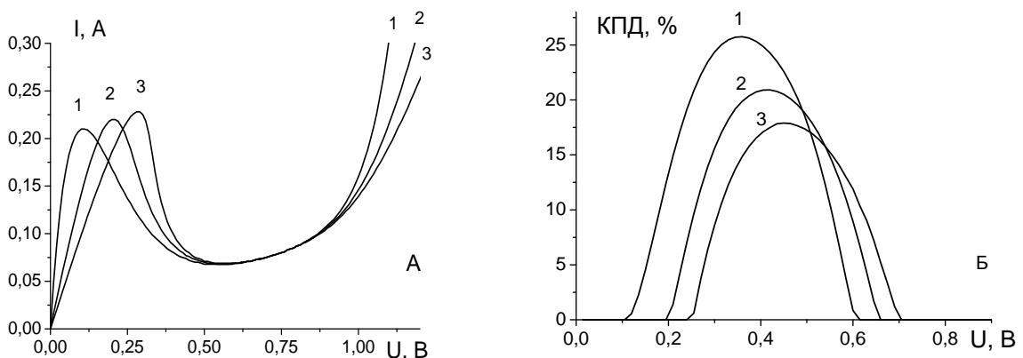
Рис.3. Вольтамперные характеристики (А) и эффективность генерации (Б): при прямом включении диода с ТГ при R 1 =10 Ом и различных R 2 : 1 – 0,01 Ом, 2 – 0,5 Ом, 3 – 0,9 Ом.
